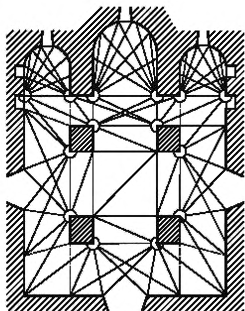
Рисунок Б.1 — Схема обмера плана методом триангуляции
