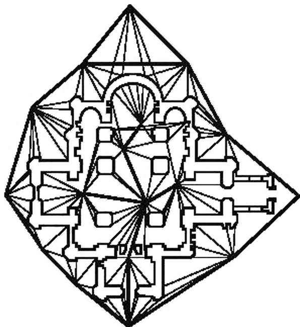
Рисунок Б.3 — Схема обмера плана с применением теодолита
