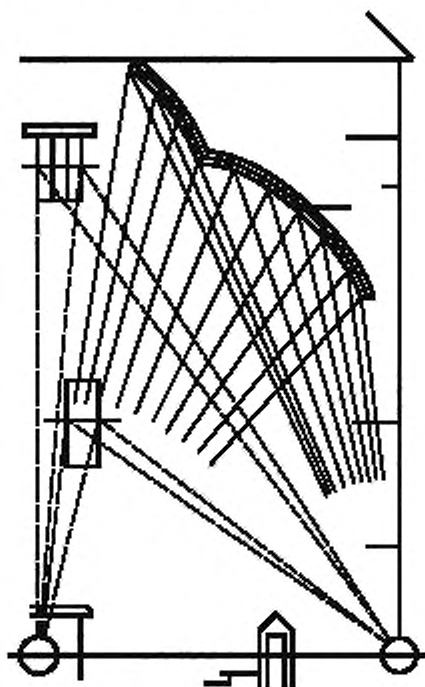
Рисунок Б.4 — Схема обмера арки от двух точек
