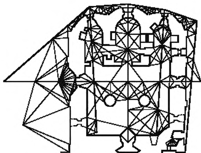
Рисунок Б.2 — Схема обмера плана с причалками
